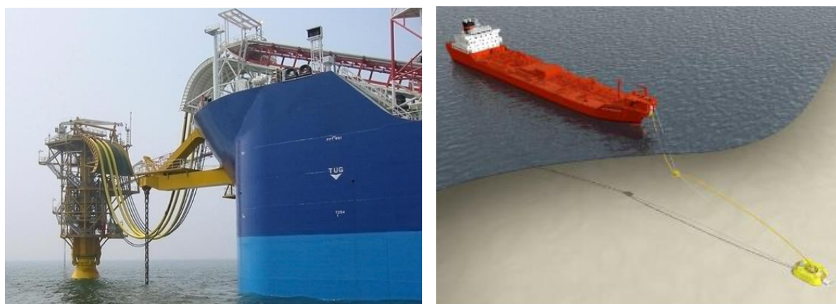
Figur 4-3: Venstre: Plattformbasert løsning Ref./27/. Høyre: Single Anchor Loading (SAL) Ref./28/
