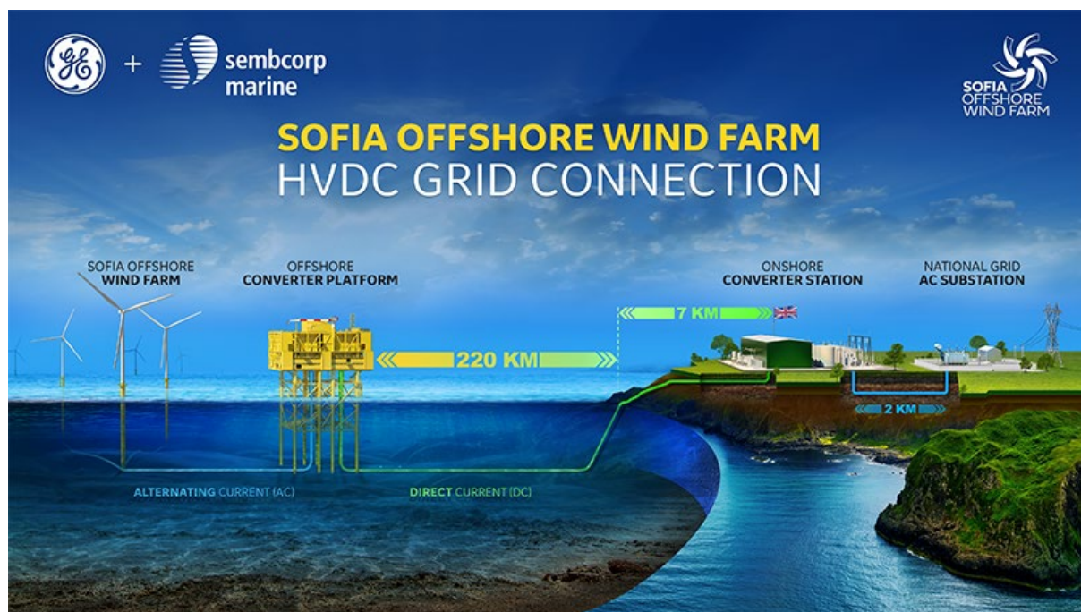
Figur 3-8 Typisk konfigurasjon for overføring av kraft til land via HVDC. Kilde: Sofia Offshore Wind Farm
